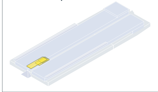
Locator map
